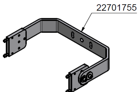
U-Arm für LA4050 mit Schenkellänge 265mm U-arm for LA4050 with arm length 265mm
