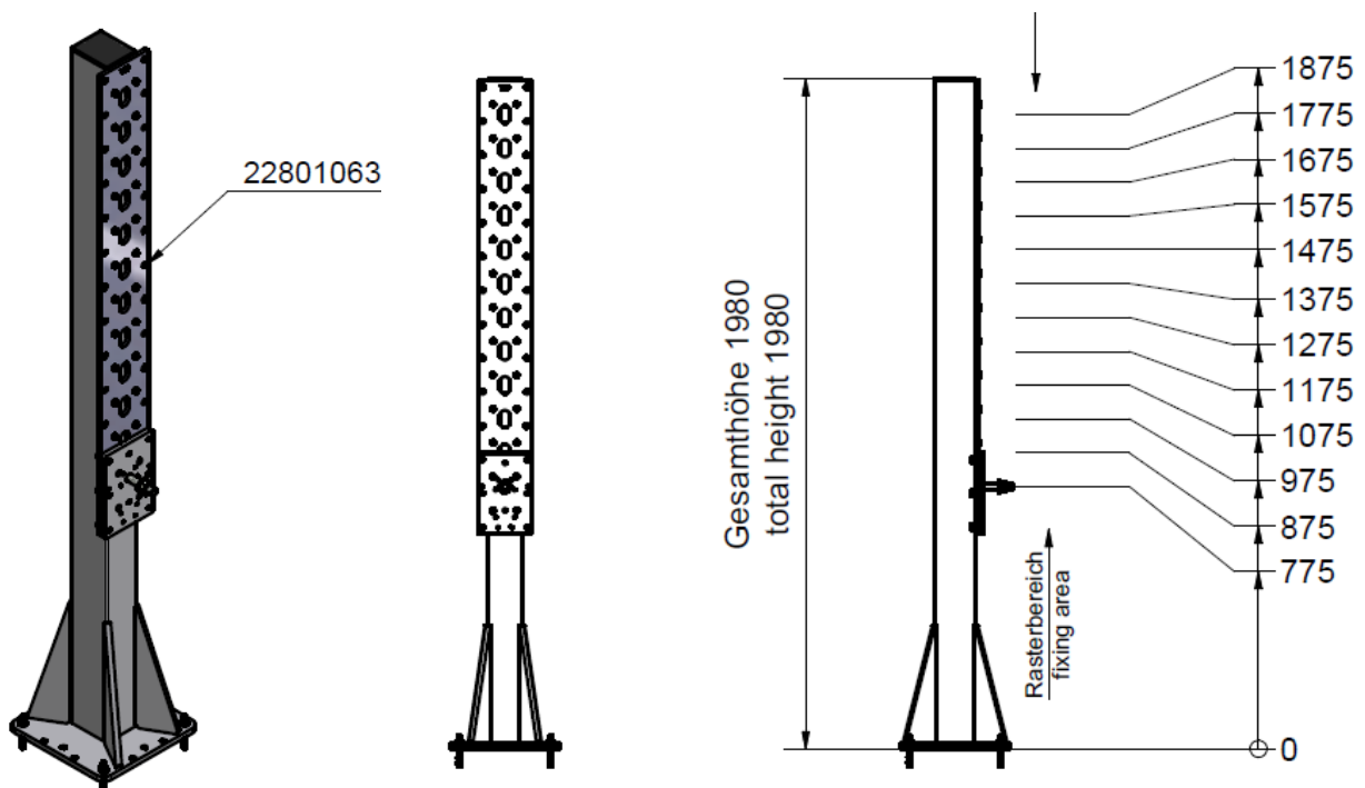
Stativ mit Fußplatte Basis Größe 2 [1980] Stand base plate basic size 2 [1980]
