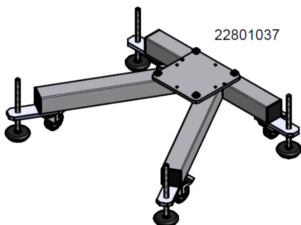
K-Fuß mit Tellerfüßen und Rollen K-foot with rubber feet and rolls
