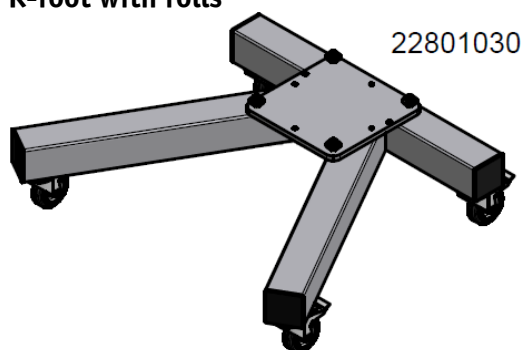
K-Fuß mit Rollen K-foot with rolls
