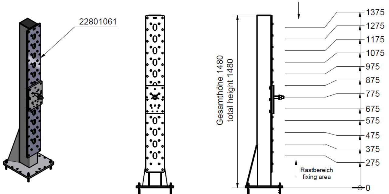
Stativ mit Fußplatte Basis Größe 1 [1480] Stand base plate basic size 1 [1480]
