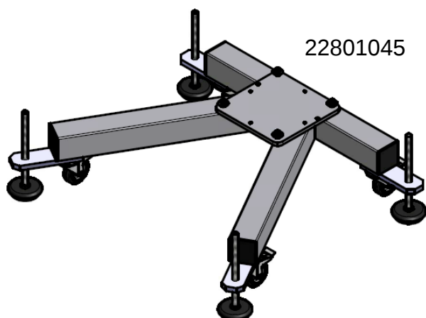
K-Fuß VA mit Tellerfüßen und Rollen K-foot SS with rubber feet and rolls
